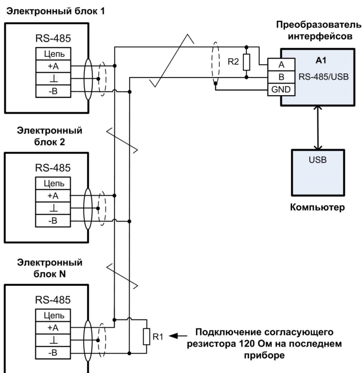
Рисунок Г.5 – Подключений нескольких блоков в локальной сети по интерфейсу RS-485 к компьютеру (или системе АСУ) при работе на длинную линию: согласующие резисторы R1, R2 – C2-33м-0,25-120 Ом \pm 5\%
