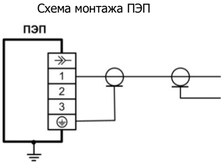
Рисунок Б.9 – Подключение цепей датчика ПЭП
