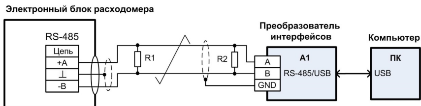
Рисунок Г.4 – Схема подключений интерфейса RS-485 к компьютеру (или системе АСУ) при работе на длинную линию: R1, R2 – C2-33м-0,25-120 Ом \pm 5\%
