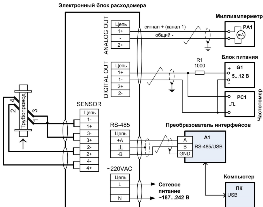
Рисунок Г.2 – Подключение одноканального расходомера при установке ПЭП на трубе по двум хордам: G1 – стабилизированный блок питания, преобразующий переменное сетевое напряжение 220 В в постоянное 12 В (выходной ток до 100 мА); PA1 – миллиамперметр на ток 4–20 мА (или вход контроллера АСУ); PC1 – частотомер на диапазон 0–2000 Гц (или вход контроллера АСУ); A1 – преобразователь интерфейсов RS-485/USB любого типа; ПК – персональный компьютер
