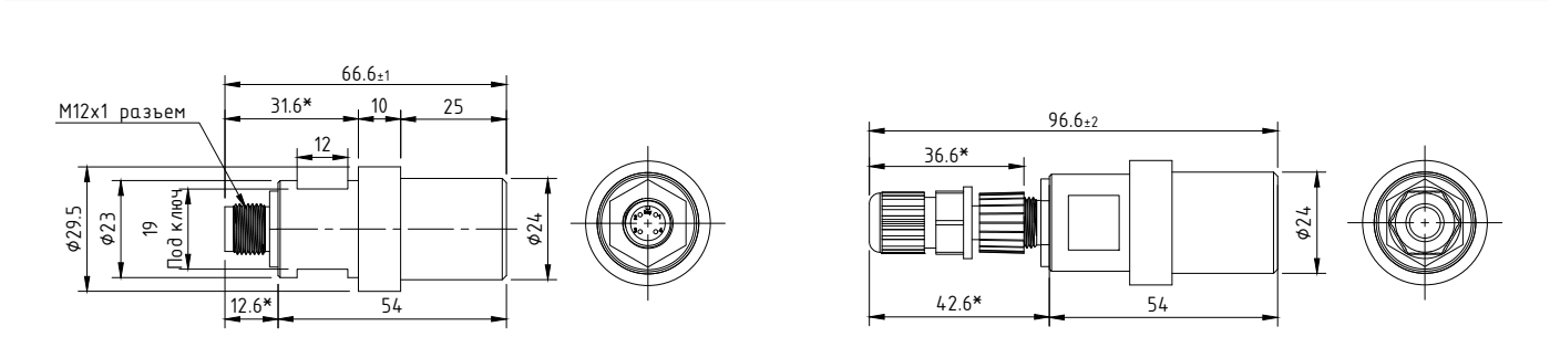
с разъемом M12x1 (IP67)
