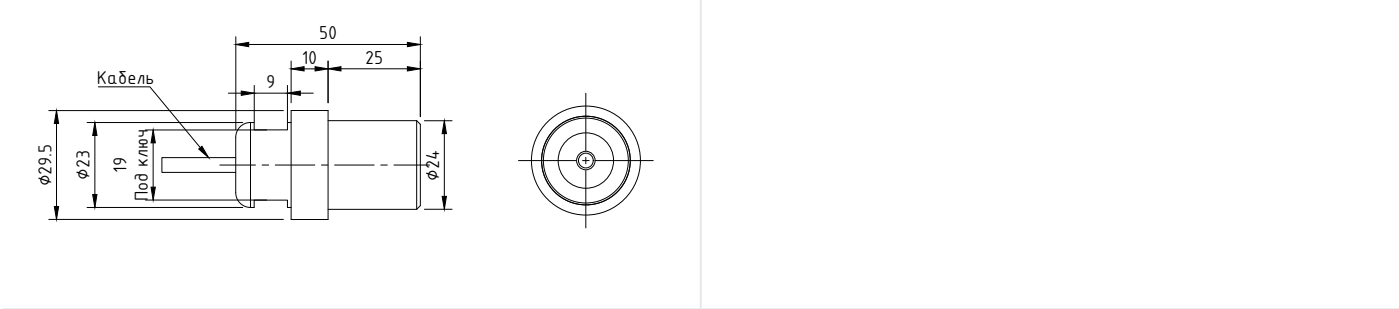
с кабельным вводом (IP68)
