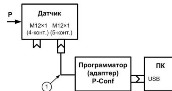
Рисунок Б.1 – Подключение программатора: 1 – встроенный в программатор кабель, P – измеряемое давление
