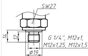
G1/4" DIN 3852
