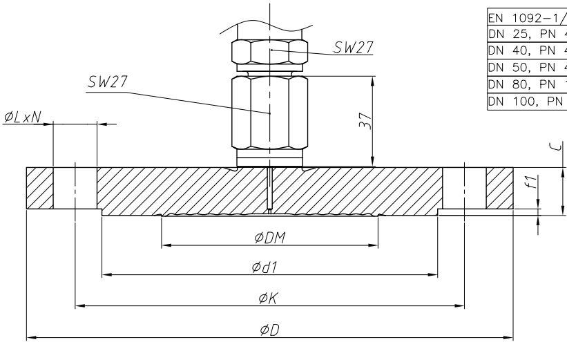
Фланцевое присоединение EN 1092-1/B
