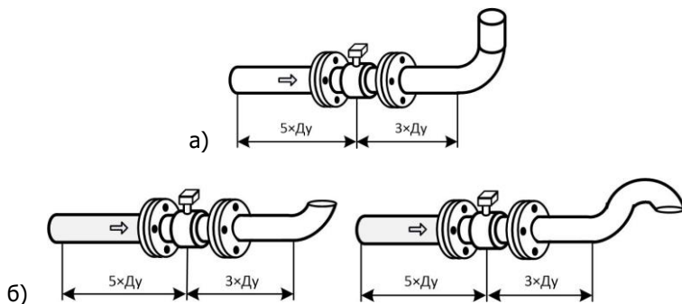
Рисунок 5.2 – Горизонтальная установка сенсора с обязательными прямыми участками на входе и выходе: а) в обычном напорном трубопроводе; б) отвод с открытым концом
