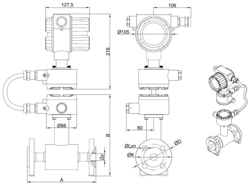
Рисунок Б.16 – Габаритные размеры взрывозащищенного расходомера (корпус 2)
