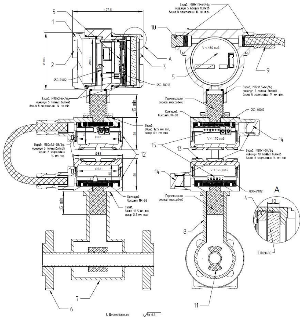
Рисунок М.4 – Особенности конструкции взрывозащищенного раздельного исполнения расходомера (корпус 2) – пояснения в таблице:
