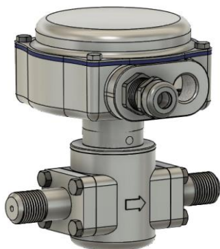
Рисунок Б.12 – Конструкция сенсора для малых диаметров Ду: а) раздельное исполнение с разъемом; б) компактное исполнение с ЭБ; в) раздельное компактное исполнение (с монтажной коробкой)
