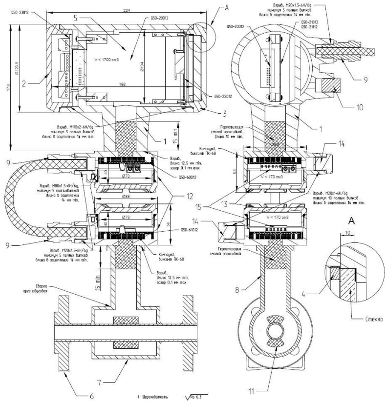
Рисунок М.3 – Особенности конструкции взрывозащитного раздельного исполнения расходомера (корпус 1) – пояснения в таблице:
