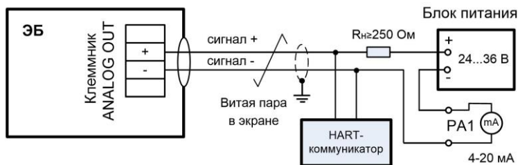
Рисунок Г.11 – Вариант подключение HART-коммуникатора
