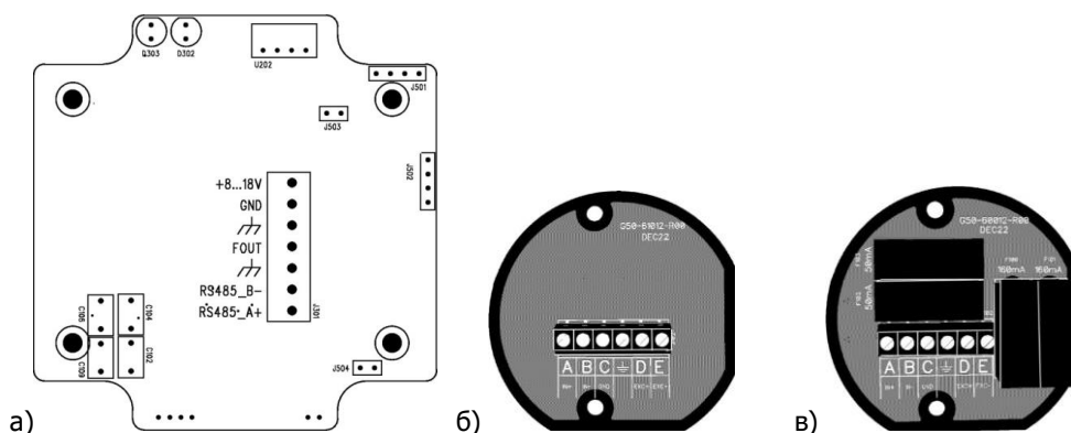
Рисунок Г.4 – Расположение контактов на клеммной колодке платы: а) для комбинированного исполнения расходомера; б) для сенсора общепромышленного исполнения; в) для сенсора
