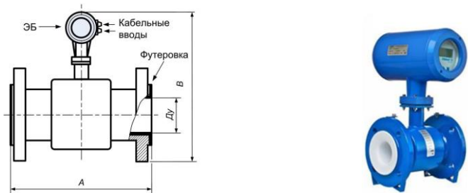
Рисунок Б.3 – Вид конструкции сенсора с установленным ЭБ
