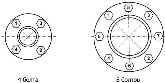
Рисунок 5.9 – Порядок затяжки или ослабления болтов крепления фланцев
