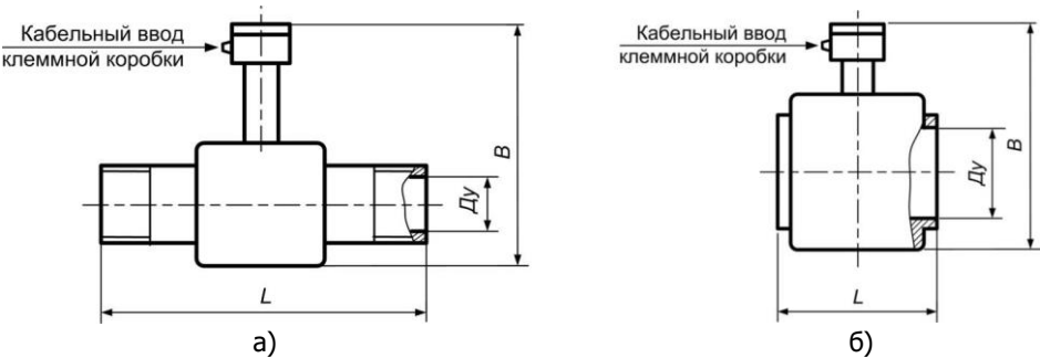
Рисунок Б.6 – Конструкция сенсора без фланцев с монтажной коробкой
