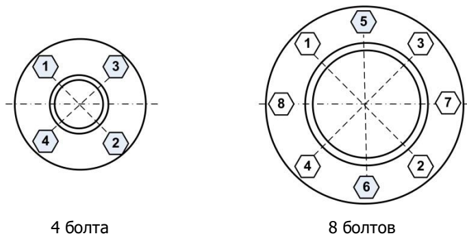
Рисунок 5.8 – Порядок затяжки или ослабления болтов крепления фланцев
