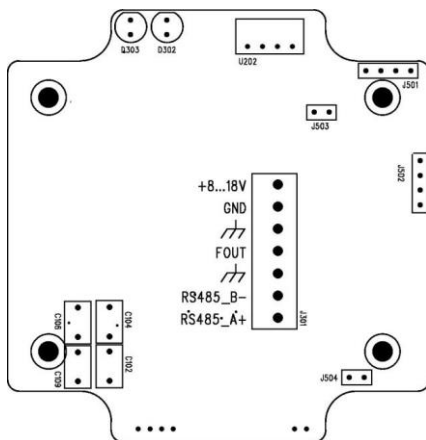
Рисунок Г.4 – В исполнении платы корпуса для термоучета показано расположение контактов на клеммной колодке
