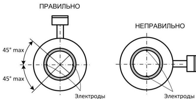
Рисунок 5.4 – Примеры положения электродов сенсора при установке
