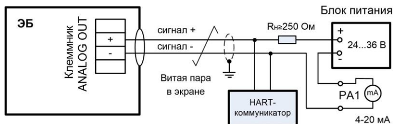
Рисунок Г.12 – Вариант подключения HART-коммуникатора
