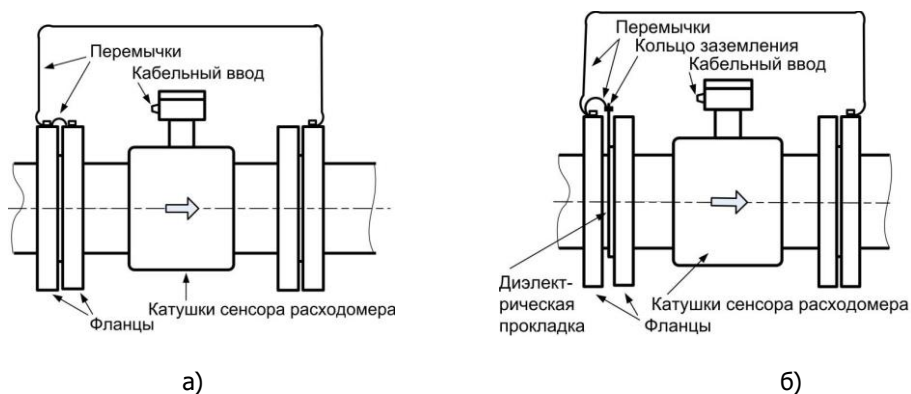
Рисунок 5.10 – Схема соединения фланцев при использовании катодной защиты (элементы крепежа на фланцах не показаны):
