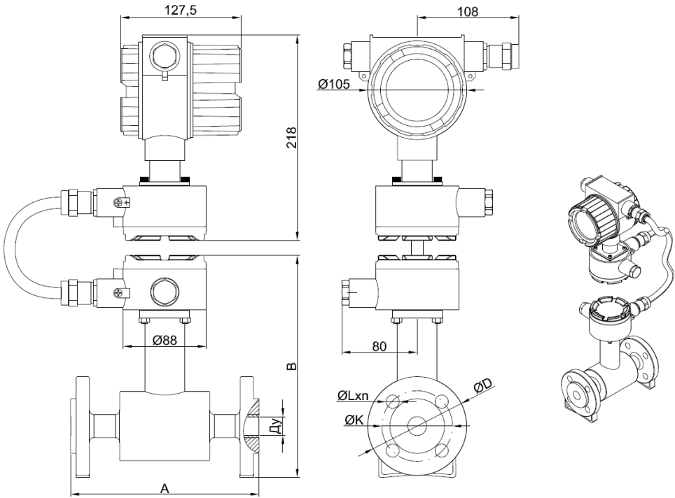
Рисунок Б.10 – Габаритные размеры взрывозащищенного раздельного исполнения (корпус 2)
