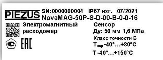
Рисунок 10.1 – Примеры идентификационных наклеек на корпусах для раздельного исполнения компонентов расходомера: а) на электронный блок; б) на датчик сенсора
