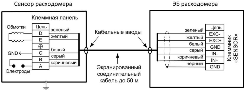
Рисунок Г.5 – Соединение сенсора с ЭБ при раздельном исполнении
