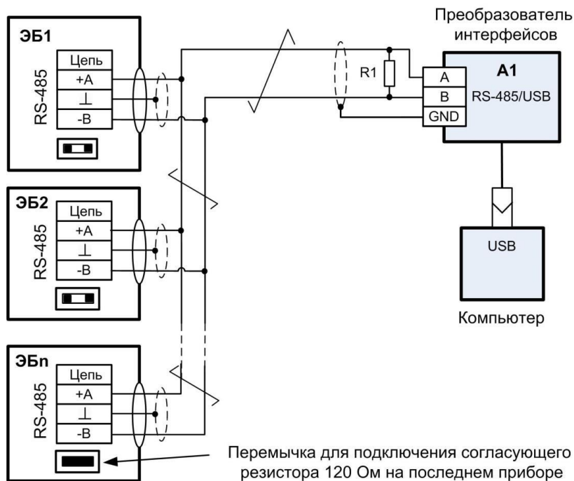
Рисунок Г.11 – Пример подключения нескольких расходомеров (или совместимых устройств) в локальной сети по интерфейсу RS-485 к компьютеру (или системе АСУ ТП) при работе на длинную линию, согласующий резистор R1 – 120 Ом \pm 5\%
