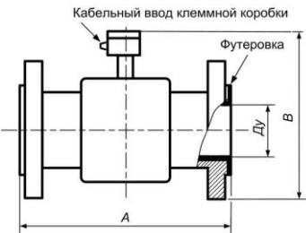
Рисунок Б.5 – Проточная часть раздельного исполнения расходомера (сенсора с монтажной коробкой, невзрывозащищенного)
