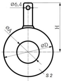
Рисунок Б.10 – Габаритные размеры заземляющих дисков (колец) для фланцевых соединений с Ду от 700 мм (A, D, H – размеры для справок)
